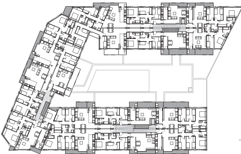
PLANTA primera E 1:600
