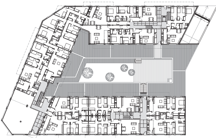
PLANTA baixa E 1:600
