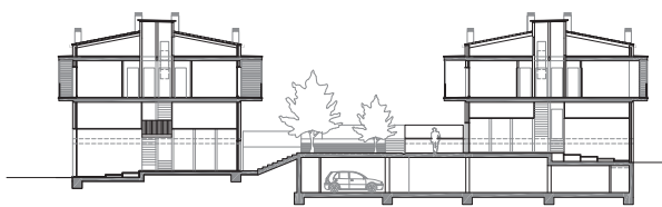
SECCIÓ transversal2 E 1:600
