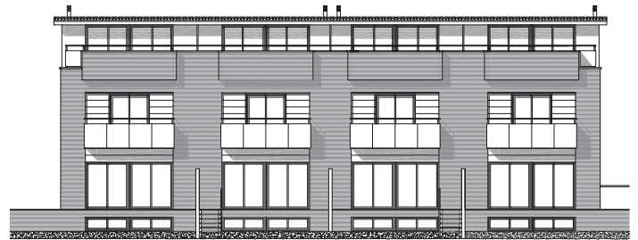
ALÇAT SUD E 1:300
