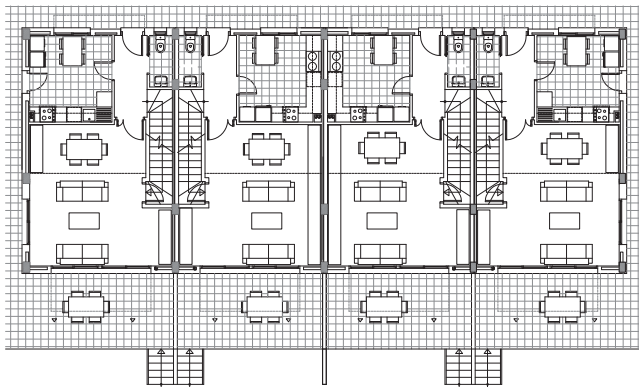
PLANTA BAIXA E 1:300
