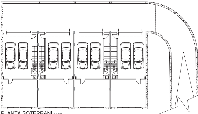
PLANTA SOTERRANI E 1:300
